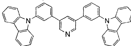
35DCzPPy
