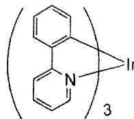
[Ir(ppy) 3 ]
