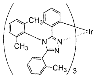
[Ir(mpptz-dmp) 3 ]
