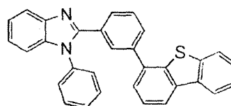
mDBTBlm-II
