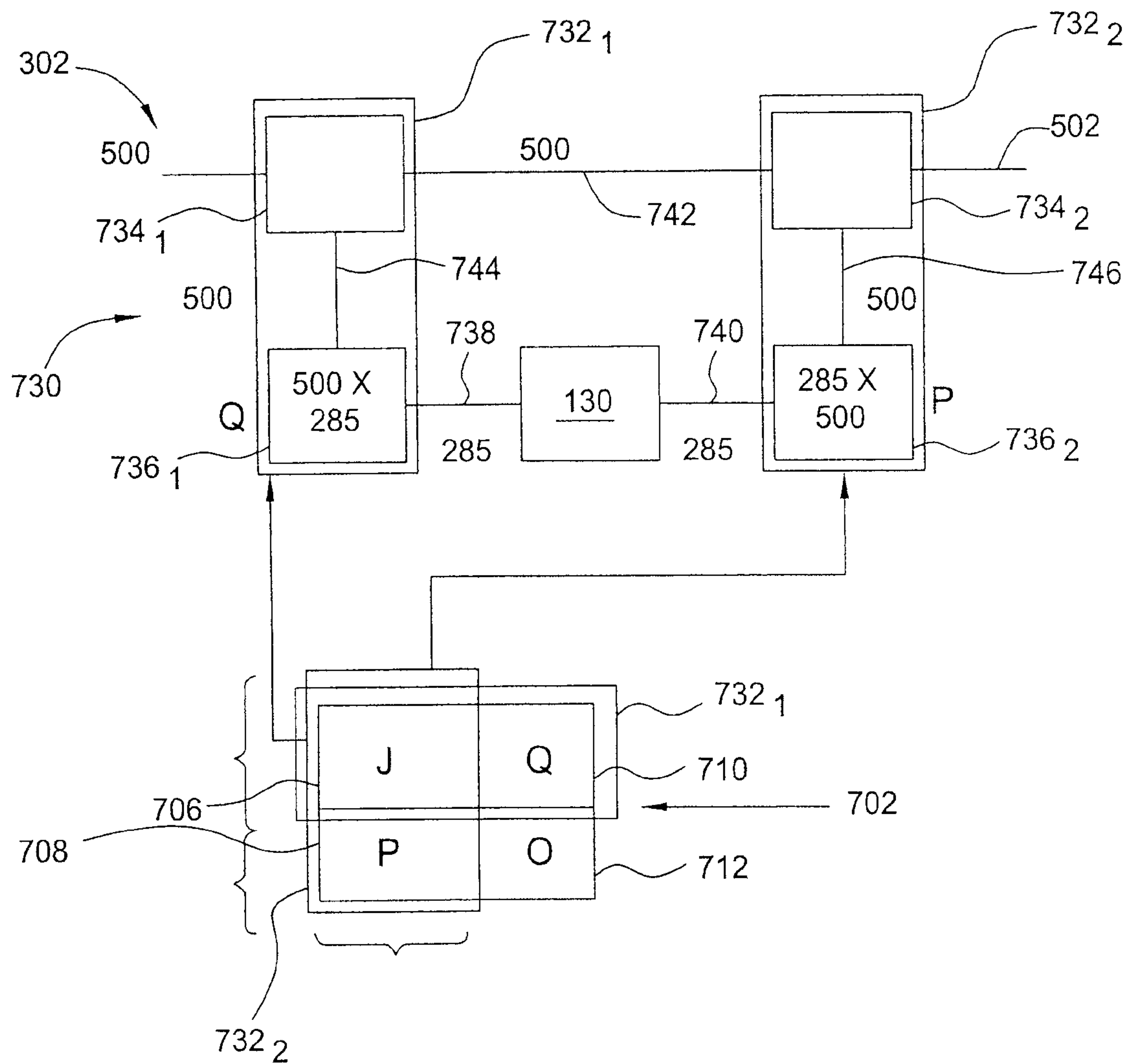
FIG. 7B
