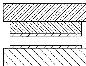
FIG. 6F
