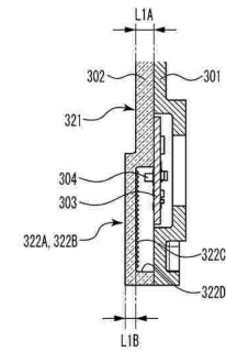
(A) 第1演出ユニット300
