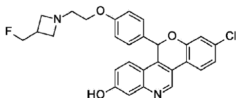
8-chloro-5-(4-{2-[3-(fluoromethyl)azetidin-1-yl]ethoxy}phenyl)-5H-[1]benzopyrano[4,3-c]quinolin-2-ol; -
