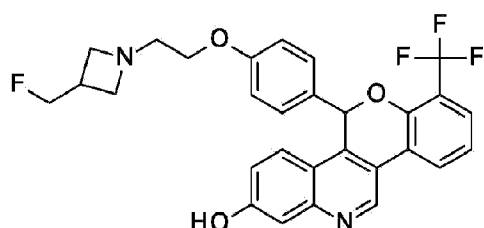
5-(4-{2-[3-(fluoromethyl)azetidin-1-yl]ethoxy}phenyl)-7-(trifluoromethyl)-5H-[1]benzopyrano[4,3-c]quinolin-2-ol;
