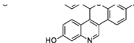
8-fluoro-5-(4-{2-[3-(fluoromethyl)azetidin-1-yl]ethoxy}phenyl)-5H-[1]benzopyrano[4,3-c]quinolin-2-ol; -
