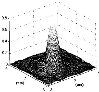
Coma FIG. 5C
