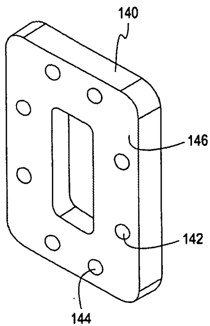
FIG. 7c
