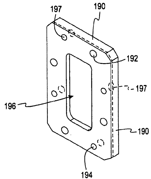
FIG. 8d
