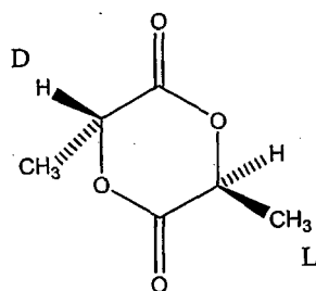
meso -D,L-lactide
