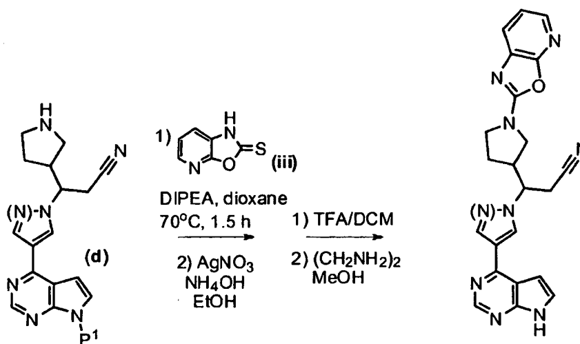
Scheme VI
