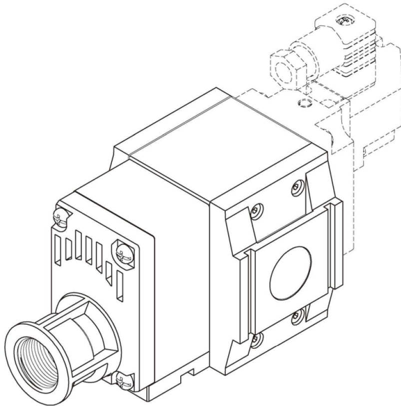
【立體圖 1】
