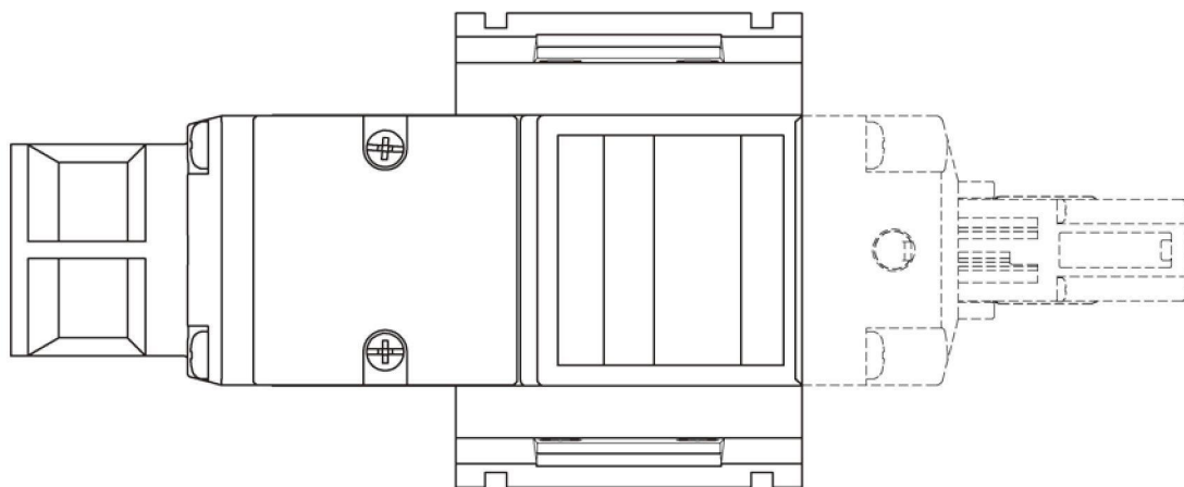
【仰視圖】
