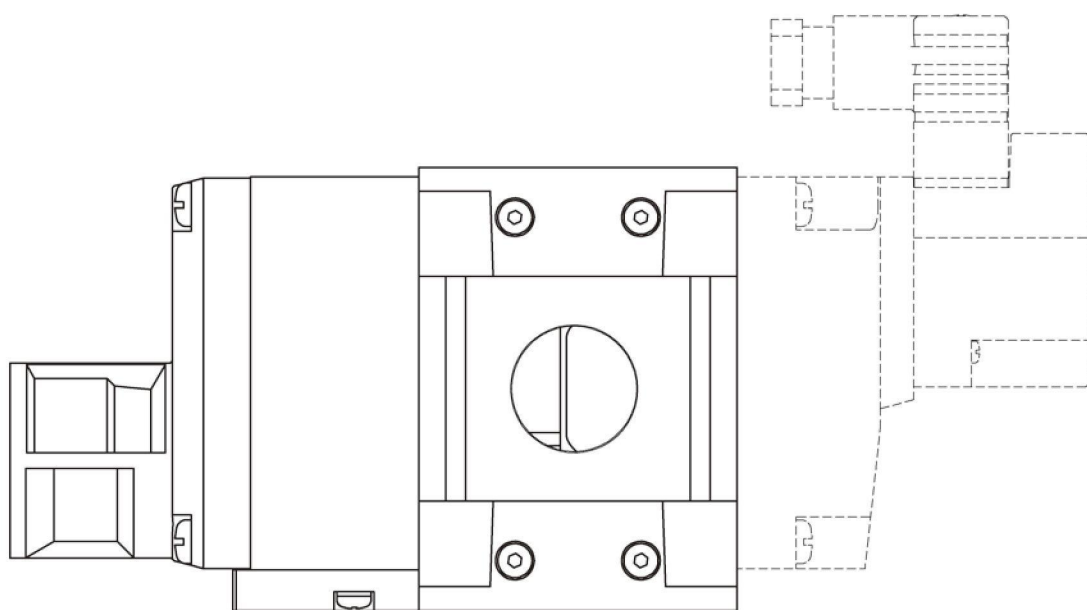
【前視圖】
