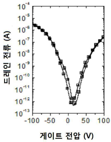
(a) 드레인 전압 = -60 V
