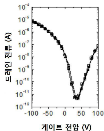
(b) 드레인 전압 = +60 V
