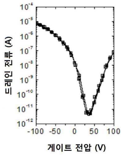
(b) 드레인 전압 = +60 V
