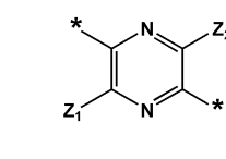
화학식 2-17
