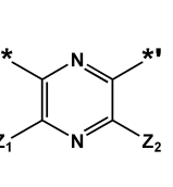
화학식 2-12
