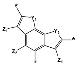
화학식 2-29
