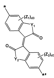
화학식 2-35
