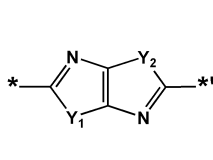
화학식 2-21
