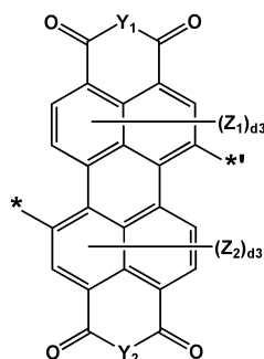
화학식 2-34
