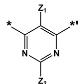
화학식 2-14
