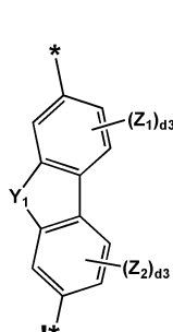
화학식 2-32
