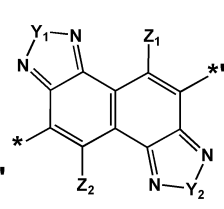
화학식 2-31
