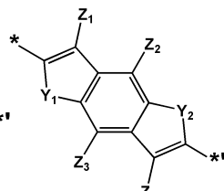
화학식 2-30
