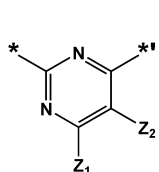
화학식 2-11
