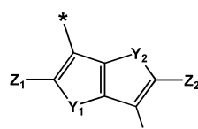
화학식 2-19
