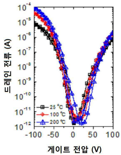
(a) 드레인 전압 = -60 V
