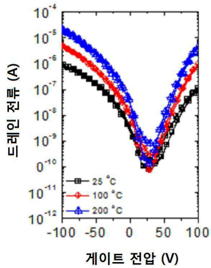
(b) 드레인 전압 = +60 V
