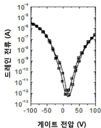
(a) 드레인 전압 = -60 V
