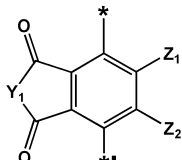
화학식 2-25
