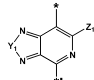
화학식 2-27
