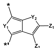
화학식 2-22
