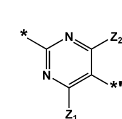
화학식 2-15
