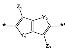
화학식 2-20
