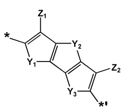
화학식 2-28
