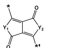
화학식 2-24
