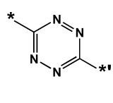
화학식 2-18
