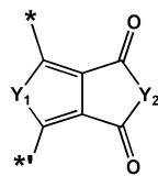
화학식 2-23
