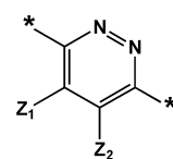
화학식 2-16
