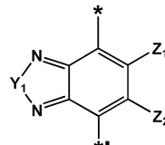
화학식 2-26
