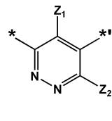
화학식 2-13
