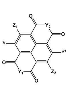
화학식 2-33
