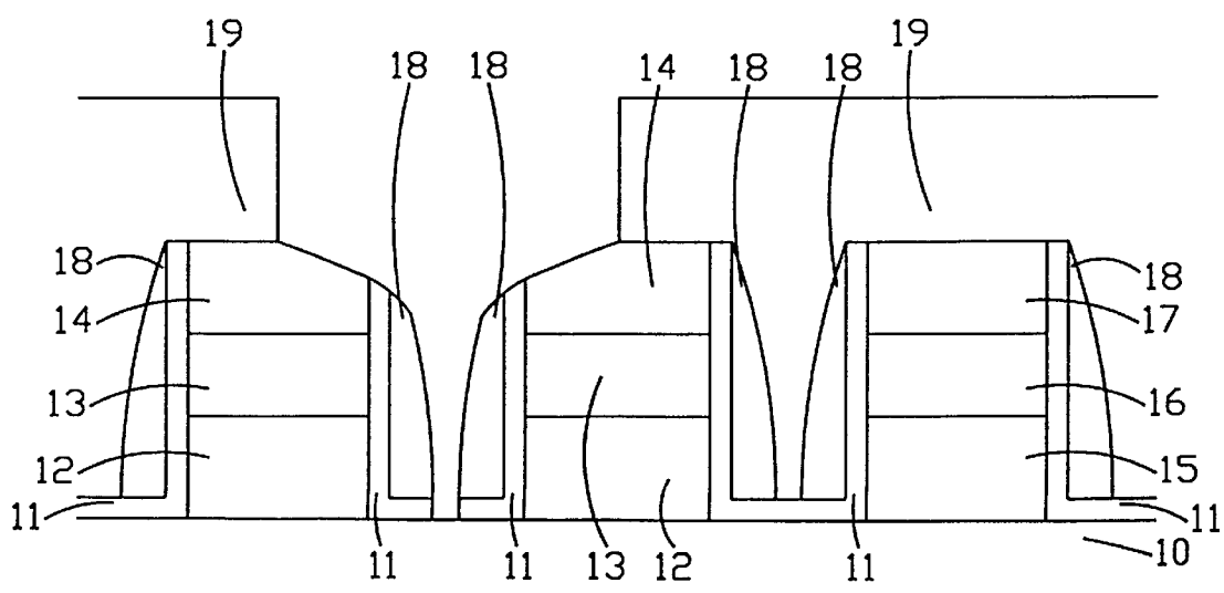
FIG.1B(Prior Art)
