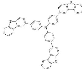
화학식 1-39'
