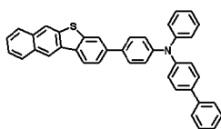
화학식 1-75'
