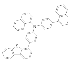
화학식 1-39'
