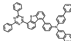
화학식 1-74'
