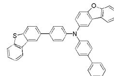
화학식 1-32'
