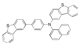
화학식 1-33'
