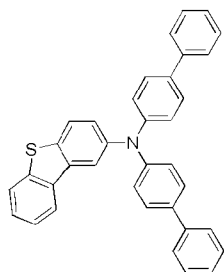
화학식 1-21'
