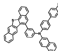
화학식 1-78'
