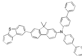
화학식 1-31'
