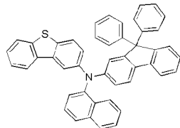
화학식 1-27'
