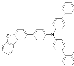
화학식 1-37'
