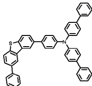
화학식 1-72'
