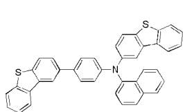
화학식 1-29'
