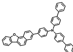
화학식 1-80'
