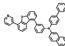
화학식 1-82'
