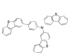
화학식 1-37'
