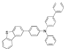
화학식 1-29'
