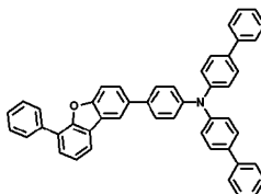
화학식 1-80'
