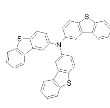
화학식 1-36'
