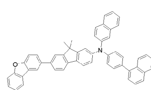
화학식 1-55'
