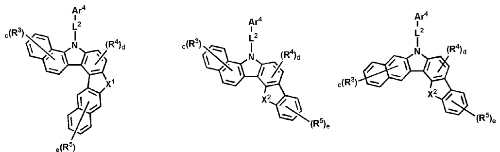
화학식 (41) 화학식 (42) 화학식 (43)
