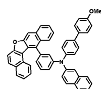
화학식 1-82'
