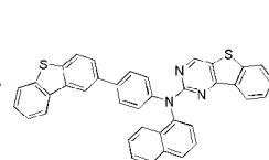
화학식 1-44'
