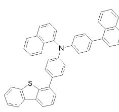
화학식 1-35'
