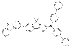
화학식 1-31'
