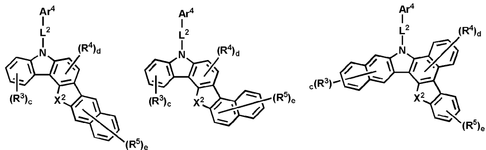
화학식 (47) 화학식 (48)
