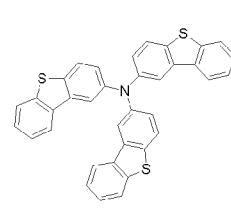
화학식 1-40'
