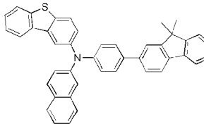
화학식 1-26'
