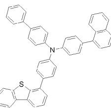
화학식 1-38'
