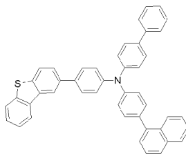
화학식 1-33'
