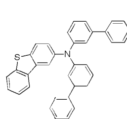
화학식 1-20'
