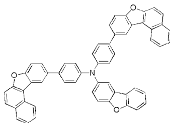
화학식 1-68'
