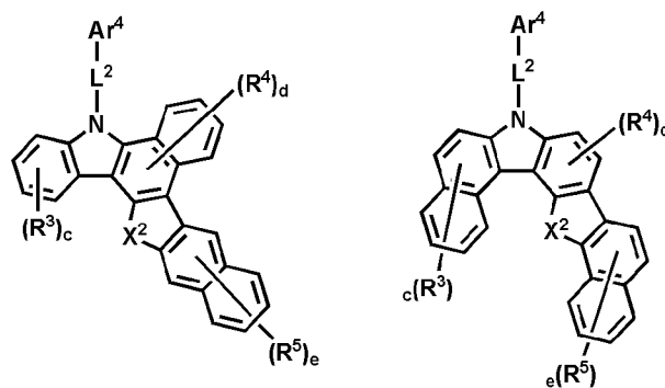
화학식 (47) 화학식 (48)
