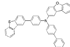
화학식 1-32'
