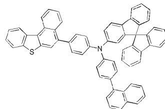
화학식 1-51'
