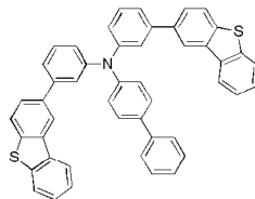
화학식 1-35'
