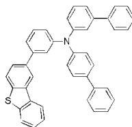
화학식 1-34'
