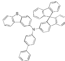
화학식 1-28'
