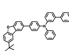
화학식 1-81'
