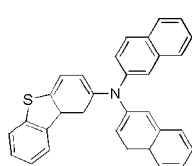
화학식 1-21'
