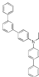
화학식 1-15'
