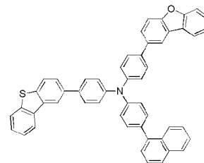
화학식 1-36'
