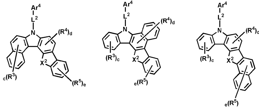
화학식 (44) 화학식 (45) 화학식 (46)
