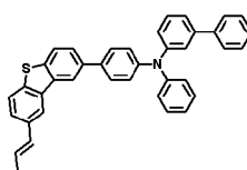
화학식 1-77'
