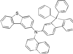
화학식 1-27'
