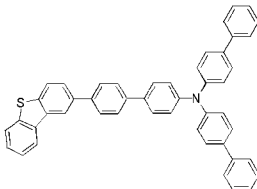
화학식 1-30'
