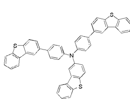
화학식 1-38'
