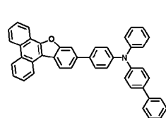
화학식 1-79'
