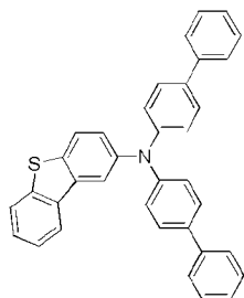
화학식 1-21'
