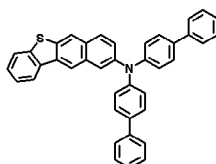
화학식 1-76'
