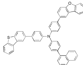
화학식 1-36'
