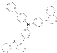
화학식 1-34'
