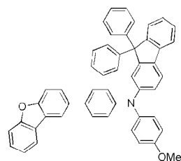
화학식 1-70'
