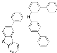
화학식 1-34'
