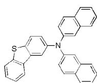
화학식 1-21'
