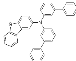
화학식 1-24'
