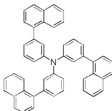
화학식 1-18'
