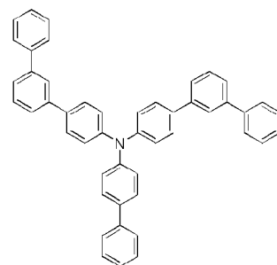
화학식 1-20'
