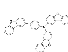
화학식 1-40'
