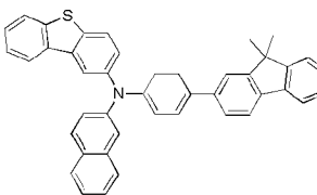
화학식 1-26'
