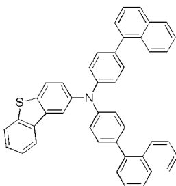
화학식 1-22'
