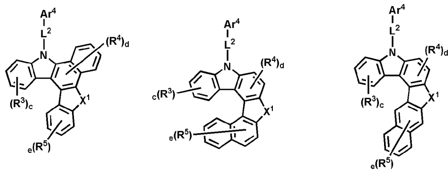
화학식 (35) 화학식 (36) 화학식 (37)
