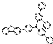
화학식 1-79'
