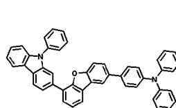
화학식 1-77'
