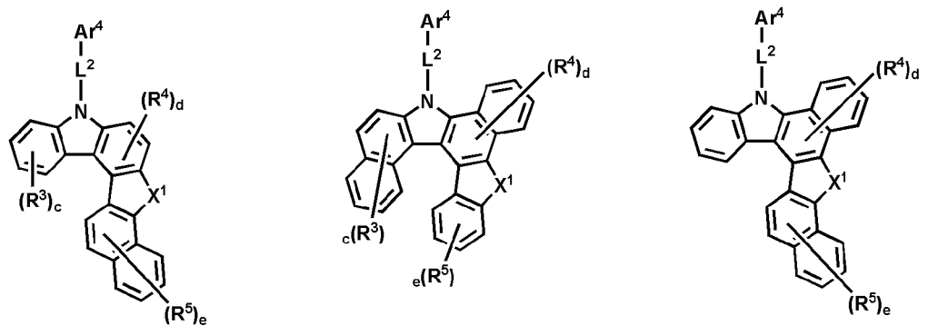
화학식 (38) 화학식 (39) 화학식 (40)
