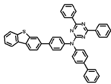
화학식 1-71'
