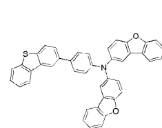
화학식 1-40'
