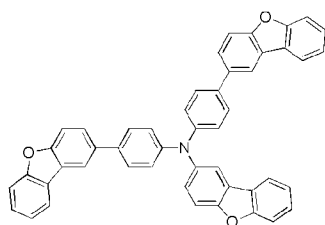
화학식 1-67'
