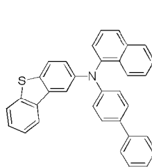
화학식 1-19'
