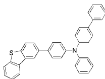
화학식 1-29'
