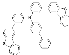
화학식 1-35'
