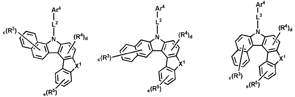
화학식 (32) 화학식 (33) 화학식 (34)
