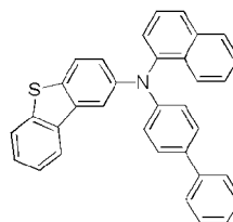
화학식 1-23'
