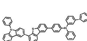
화학식 1-69'
