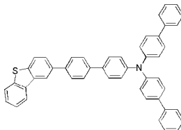
화학식 1-30'
