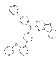
화학식 1- 59'
