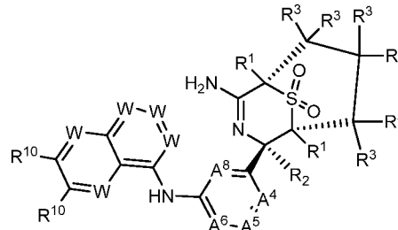
III-B-2
