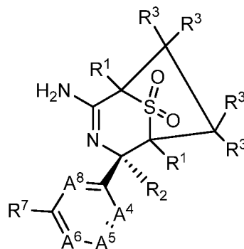
II-C
