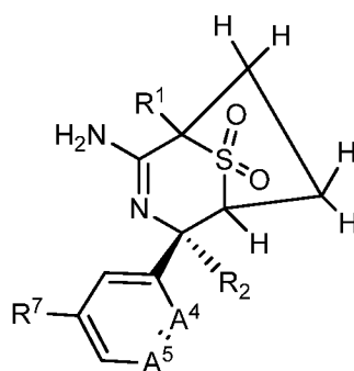
II-D
