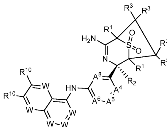
II-C-3
