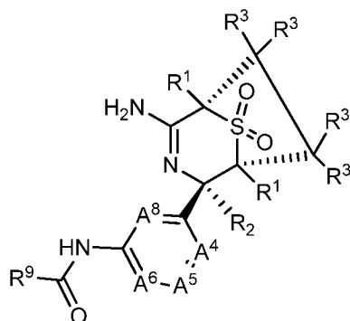
II- C-1-A
