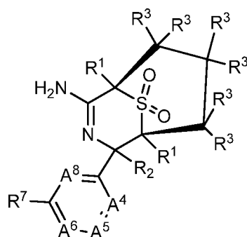
III-D
