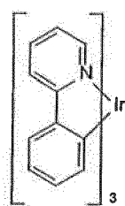
Ir(ppy) 3
