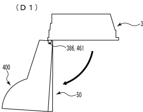
【図13-44】 開閉扉枠 [第2開状態 (開放角度: 約90度)]
