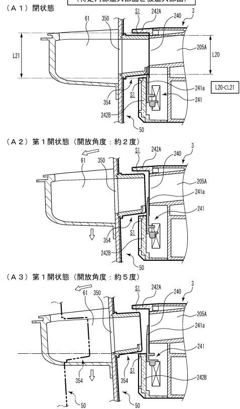
【図13-49】 抽出通路 (特定内部進入部品と被進入部品)
