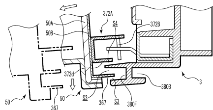
(A 3) 第1 開状態 (開放角度 : 約 5 度)
