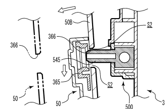
(A 3) 第1 開状態 (開放角度 : 約 5 度)
