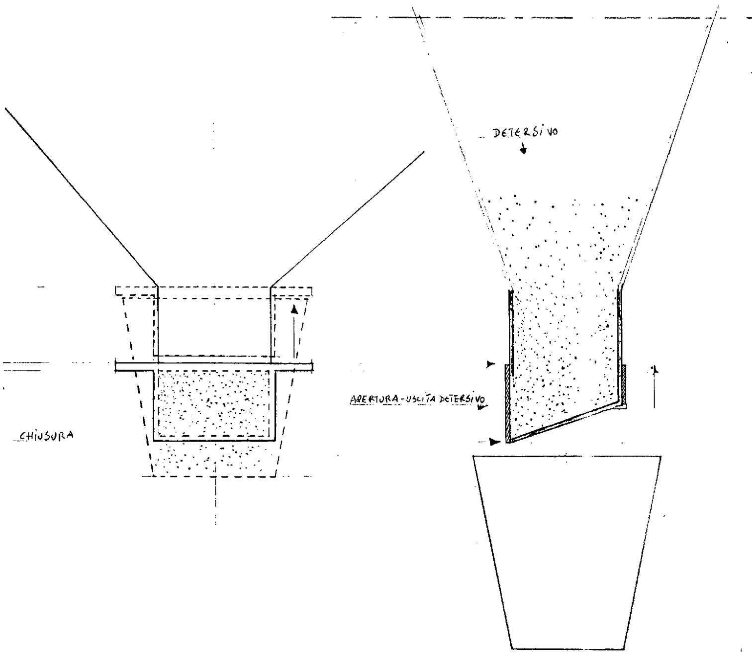
PARTICOLARE SEZ. A-A' SCALA 1:1
