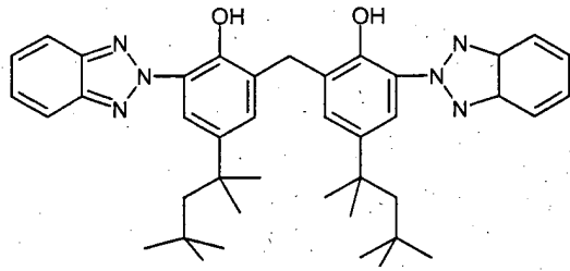
Tinuvin® 360
