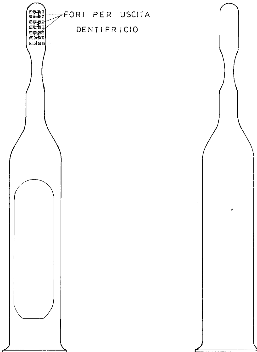
TAV. 1 Viste frontali Scala 1:1
