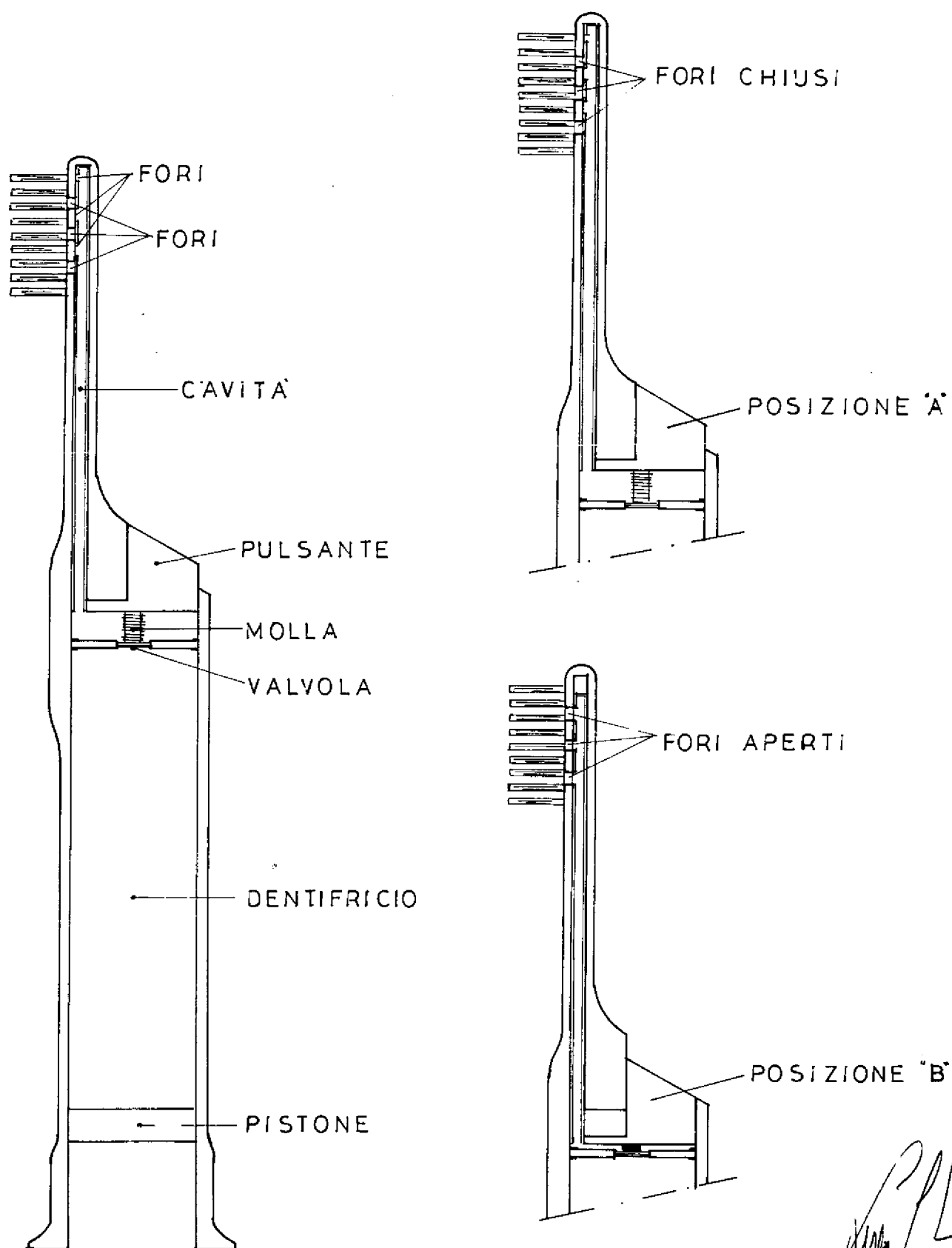
TAV. 2 Sezione e posizioni di funzionamento
