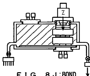
FIG. 8J: BOND
