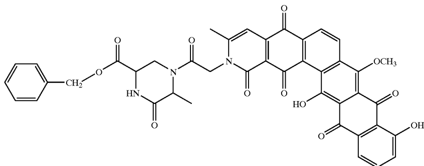
P175-A BENZYL ESTER
