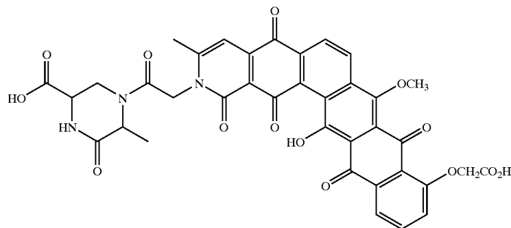
P175-A ETHER D
