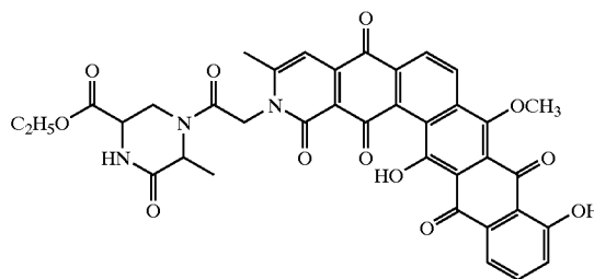
P175-A ETHYL ESTER
