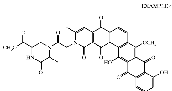
P175-A METHYL ESTER
