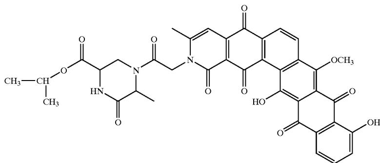
P175-A ISOPROPYL ESTER
