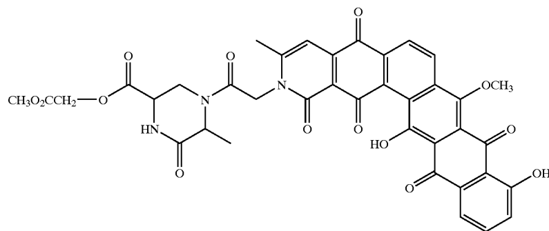
P175-A ETHER A
