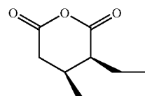
glutaric anhydride
