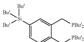
1,2-bis(di-tert-butyl(phosphino-methyl))-4-(tri-tert-butylsilyl) benzene
