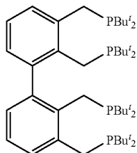
1,2-bis(di-tert-butyl(phosphinomethyl))-3-(2',3'-bis(di-tert-butyl(phosphinomethyl))phenyl)benzene
