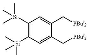
1,2-bis(di-tert-butyl(phosphino-methyl))-4,5-bis(trimethylsilyl) benzene
