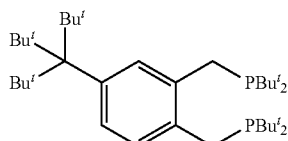
1,2-bis(di-tert-butyl(phosphino-methyl))-4-(tri-tert-butylmethyl) benzene
