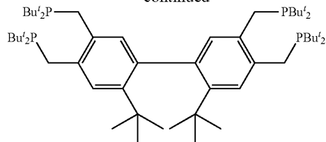
1,2-bis(di-tert-butyl(phosphinomethyl))-4-tertbutyl-5-(2'-tertbutyl-4',5'-bis(di-tert-butyl(phosphinomethyl))phenyl)benzene, and
