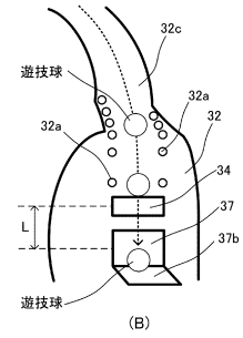
普図始動ゲートと普電の構成
