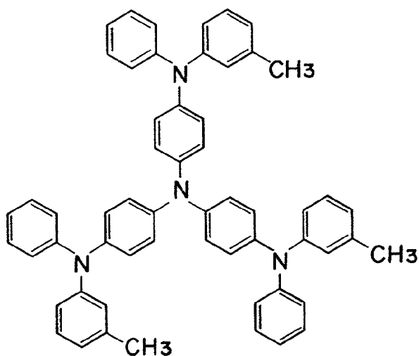
STRUCTURAL FORMULA OF m-MTDATA
