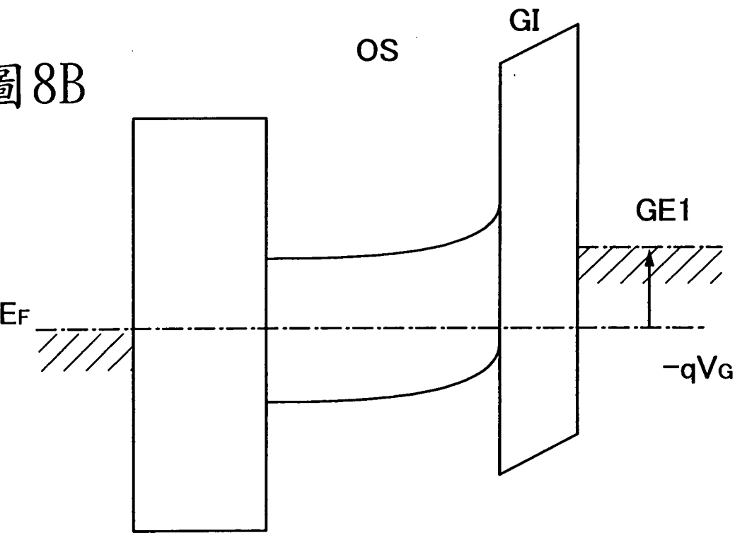
B-B'區的能量帶圖 ( V_G < 0 )
