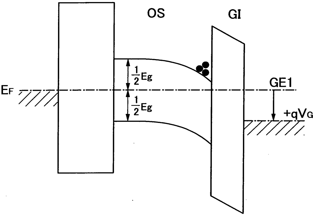
B-B'區的能量帶圖 ( V_G > 0 )
