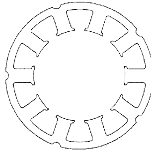
[FIG. 7(d)] 10 SLOTS (10 POLES)
