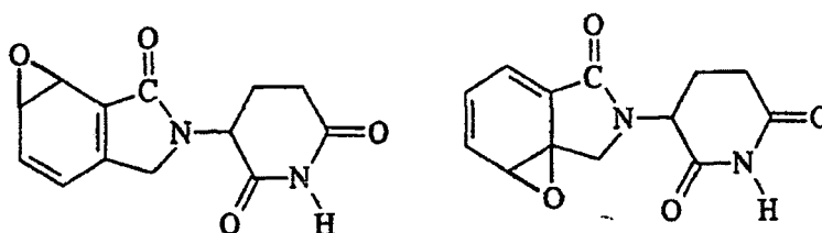
Epoxides of EM 12
