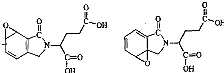
Epoxides of EM 138
