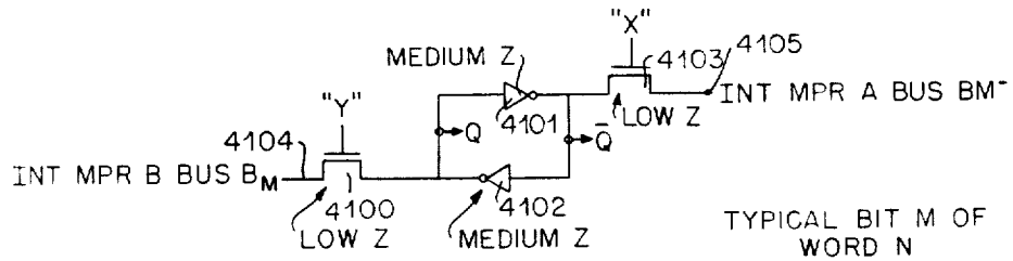
MPR FIG. 20 A. NO ALTERNATE INPUTS
