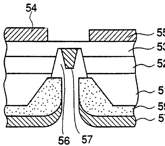
Fig.11 (d) Prior Art
