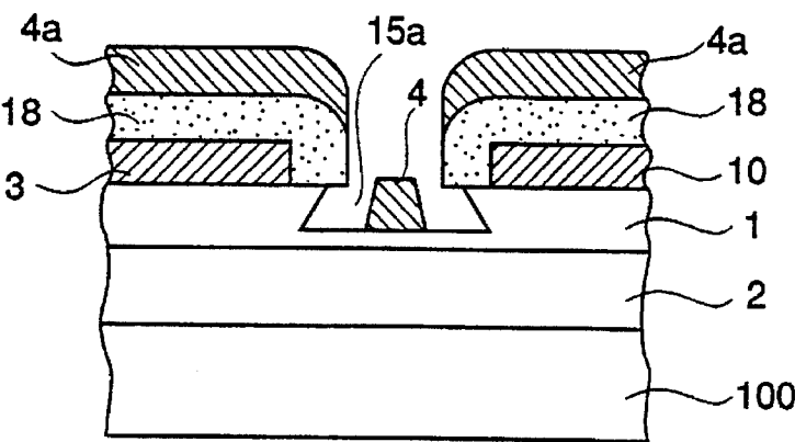
Fig.9(d) Prior Art
