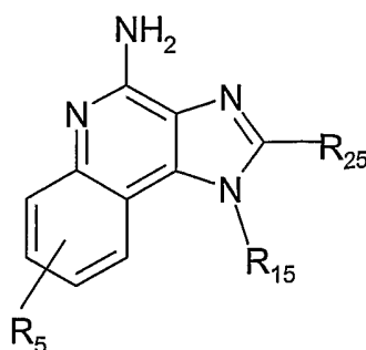
(V)
