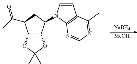
A-9
