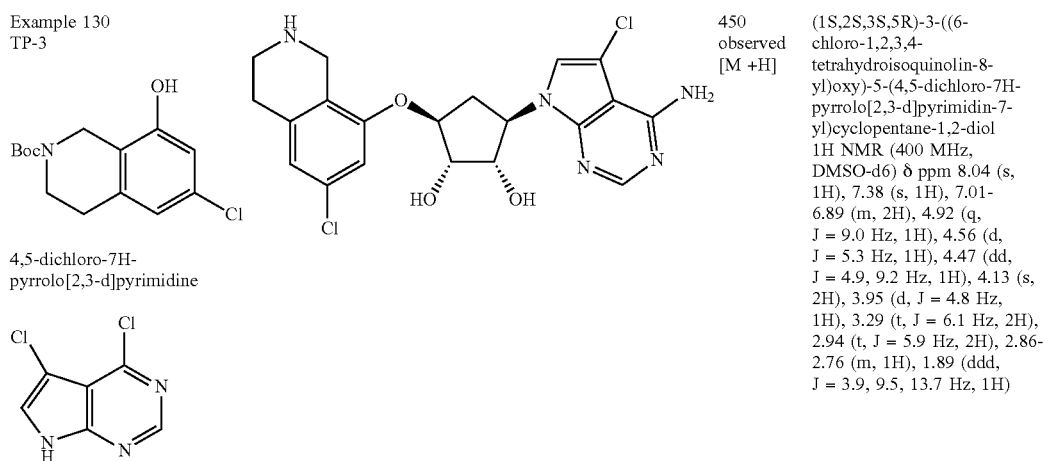
Example 131 TP-3
