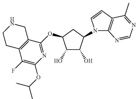
Example 193
