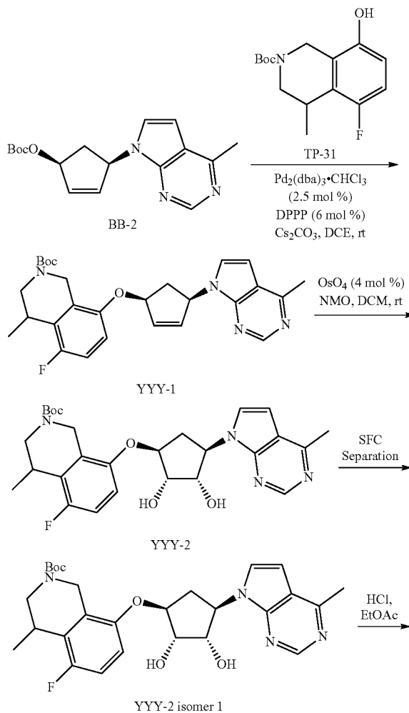
Scheme YYY
