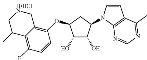
YYY-3 isomer 1
