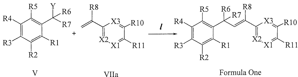
Scheme VI
