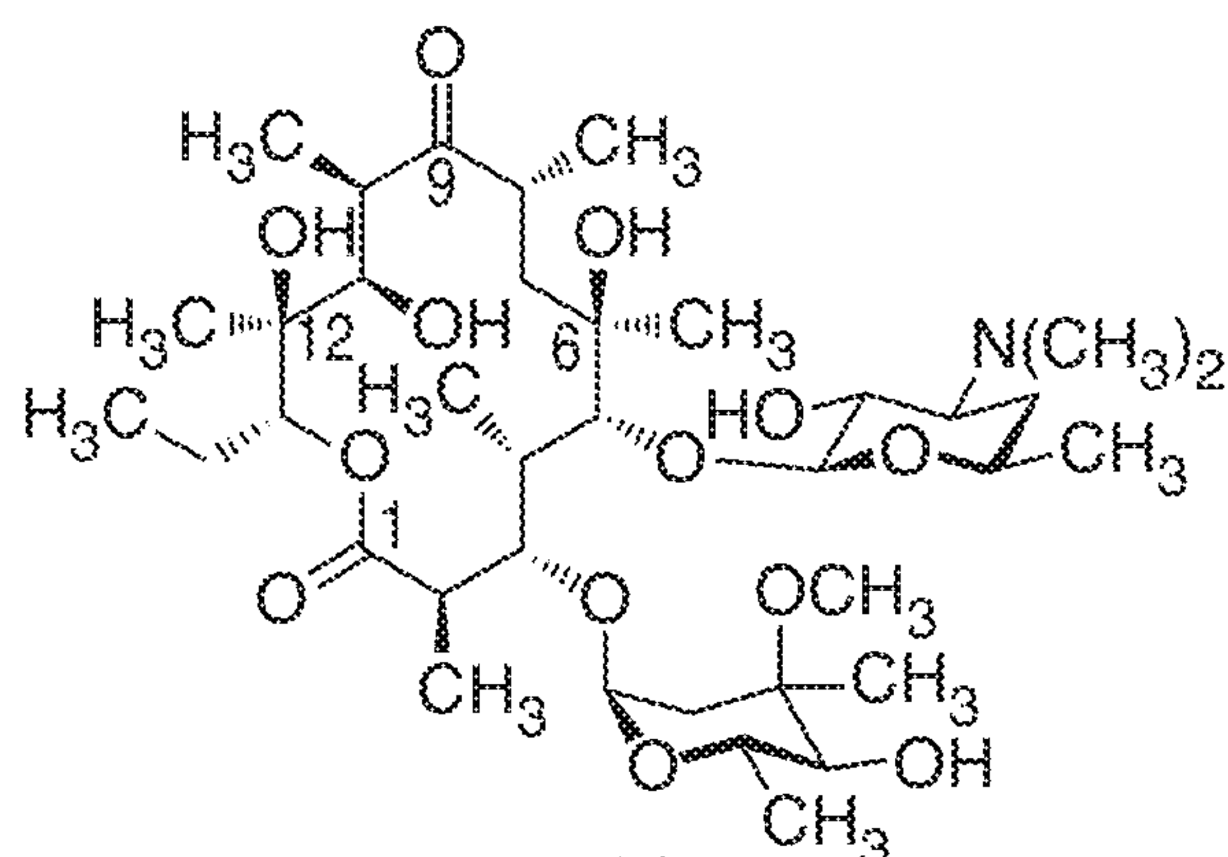
erythromycin (1)
