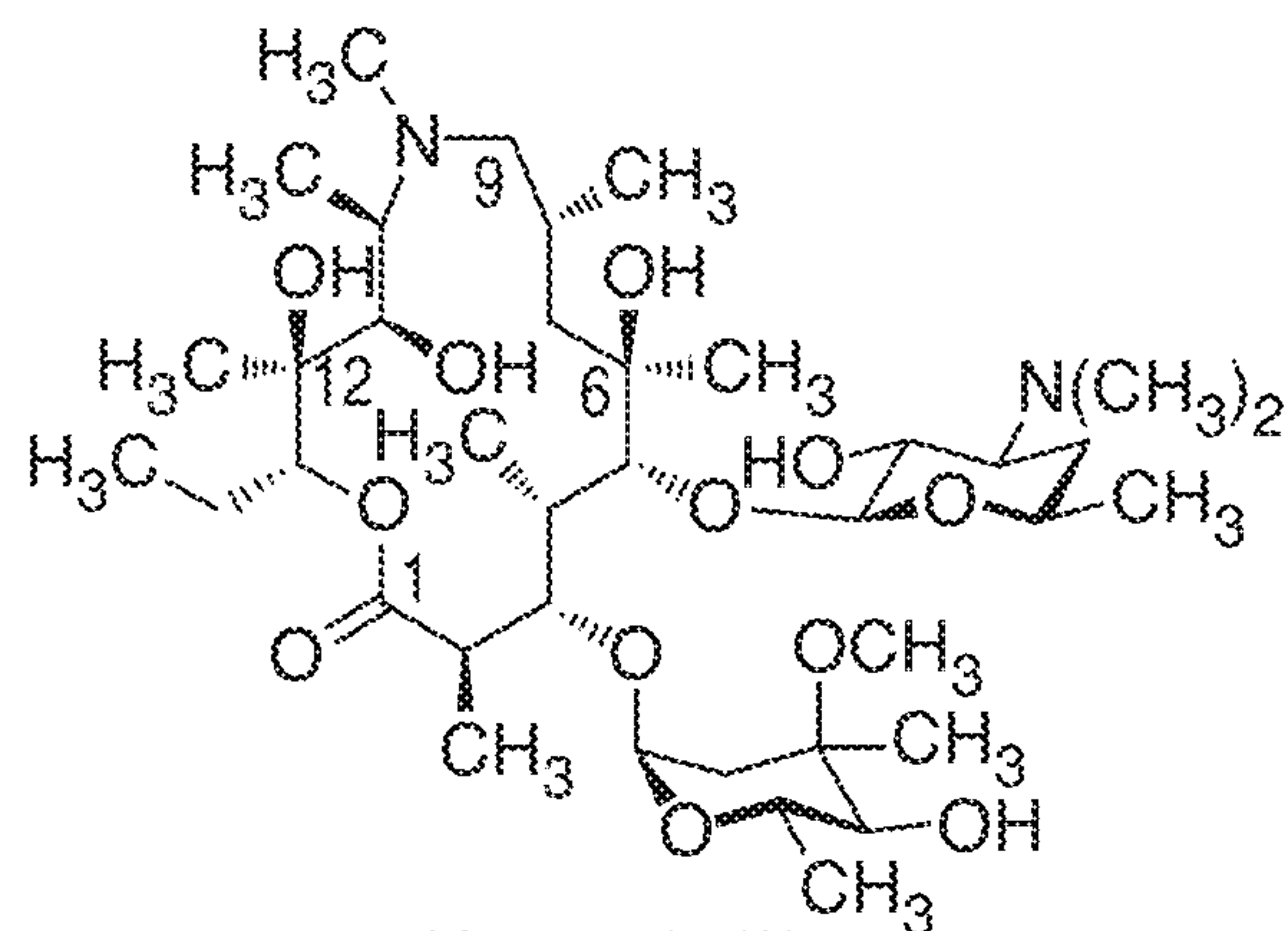
azithromycin (3)
