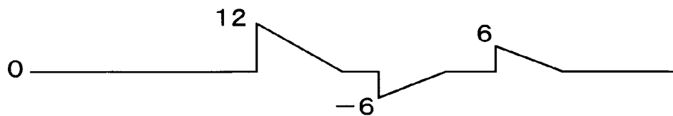
FIG.7 (d) OUTPUT OF LUMINANCE ADAPTIVE CONVERTING CIRCUIT
