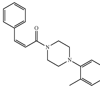
(Z)-3-Phenyl-1-(4-(o-tolyl)piperazin-1-yl)prop-2-en-1-one (14)
