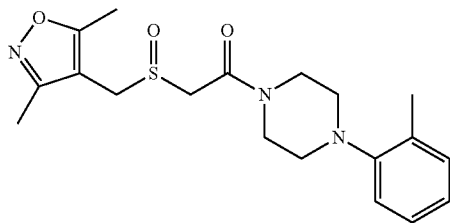
2-(((3,5-Dimethylisoxazol-4-yl)methyl)sulfinyl)-1-(4-(o-tolyl)piperazin-1-yl)ethan-1-one (12)
