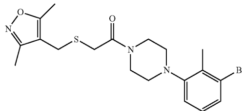
1-(4-(3-bromo-2-methylphenyl)piperazin-1-yl)-2-(((3,5-dimethylisoxazol-4-yl)methyl)thio)ethan-1-one (BRE454-75)
