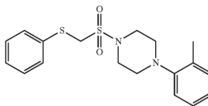
1-(((Phenylthio)methyl)sulfonyl)-4-(o-tolyl)piperazine (BRE454-84)
