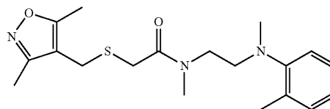
2-(((3,5-Dimethylisoxazol-4-yl)methyl)thio)-N-methyl-N-(2-(methyl(o-tolyl)amino)ethyl)acetamide (5i)
