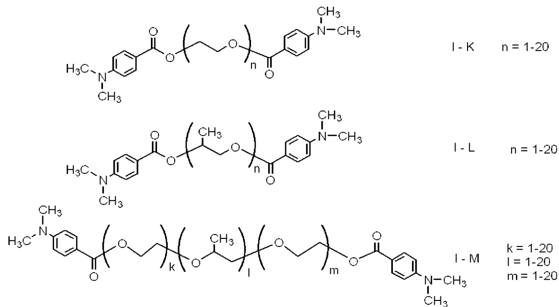
[Chem. 23]
