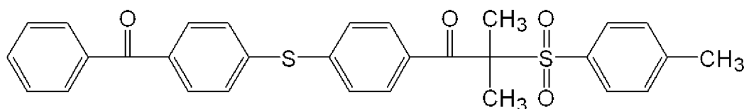
[Chem. 5]
