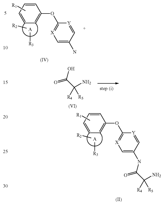
Scheme 2a
