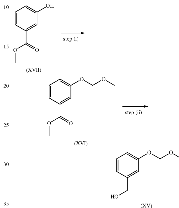
Scheme 9a
