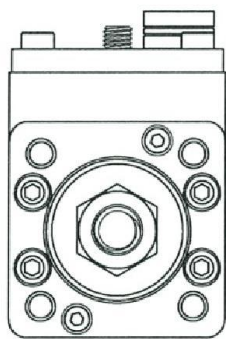
【左側視圖】
