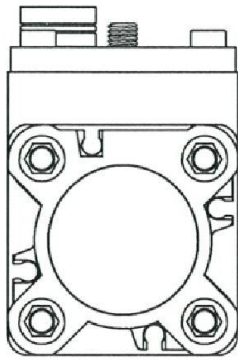
【右側視圖】
