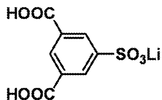
lithium 3,5-dicarboxybenzenesulfonate
