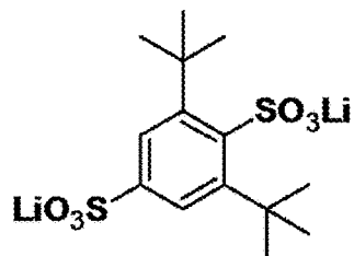
lithium 2,6-di-tert-butylbenzene-1,4-disulfonate
