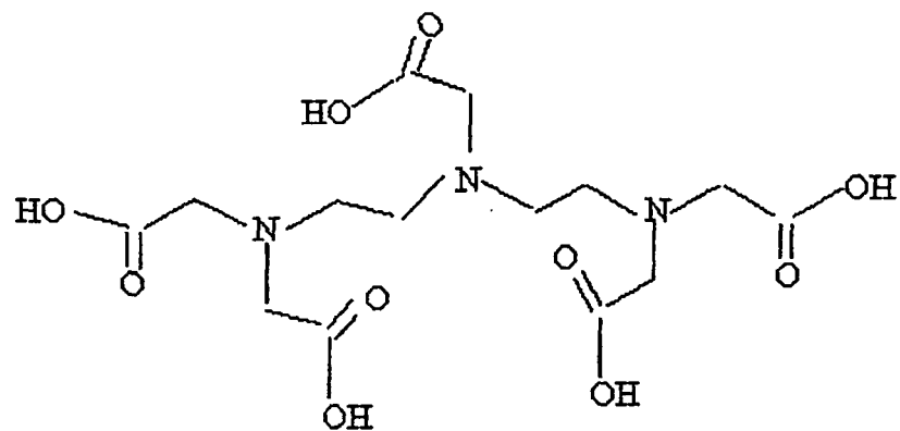
DTPA
