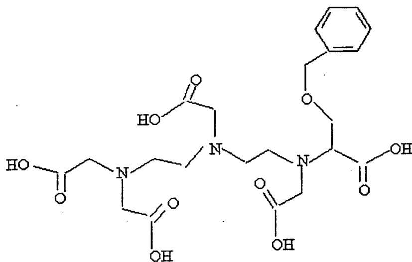
BOPTA
