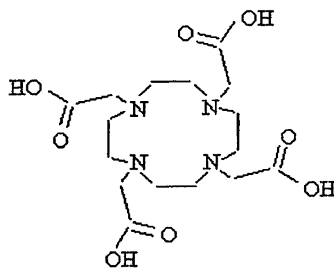
DOTA
