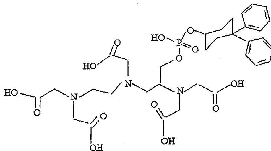
MS-325-L
