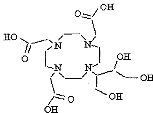
DO3A-butrol
