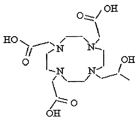
HP-DO3A
