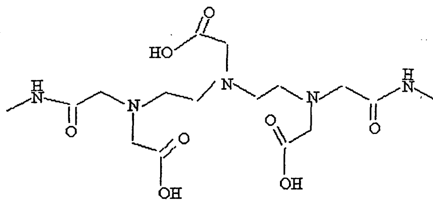
DTPA-BMA
