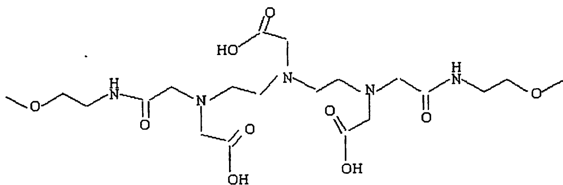
DTPA-BMEA
