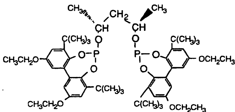
Ligand K
