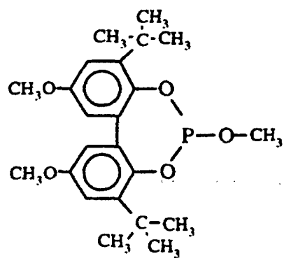
Ligand B
