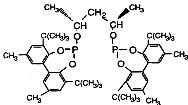
Ligand J
