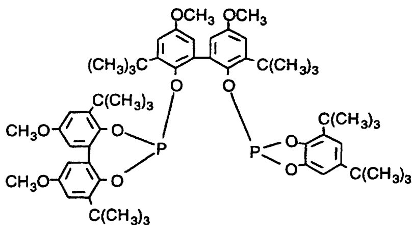
Ligand N
