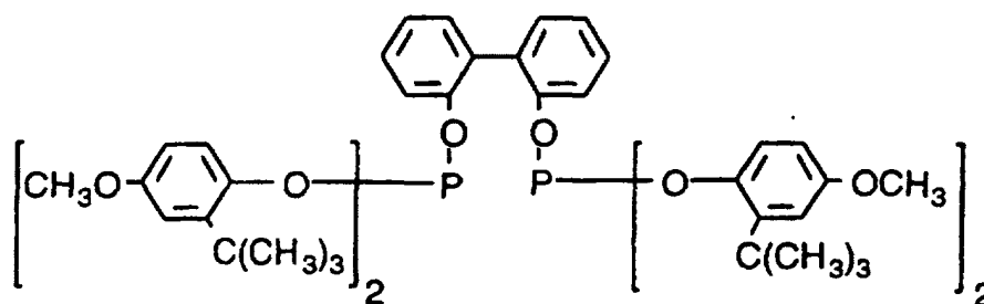
Ligand V
