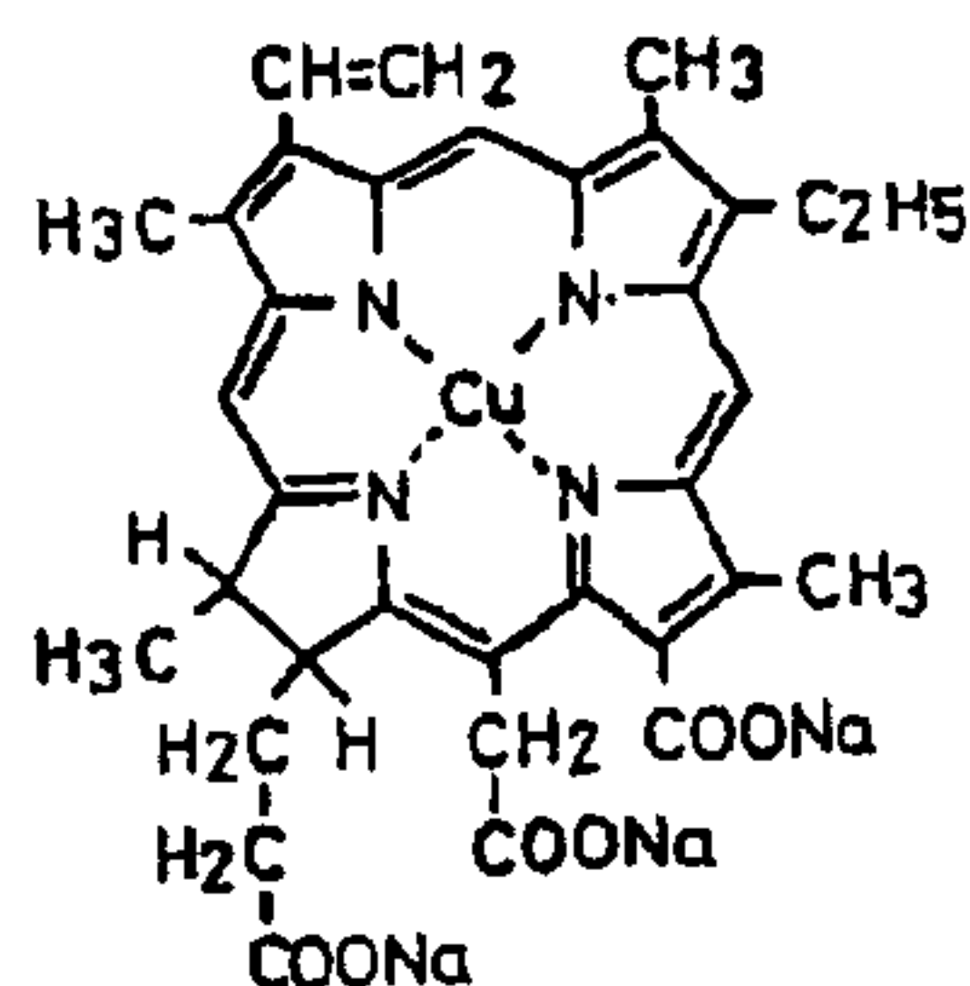
Chlorophyllin
