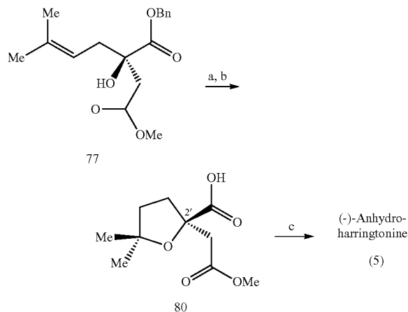
Scheme 14-1.
