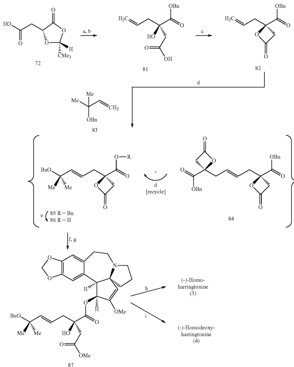
Scheme 15-1.
