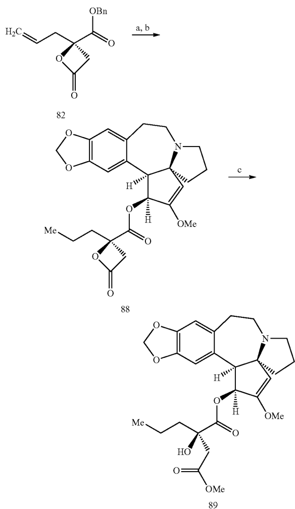
Scheme 16-1.
