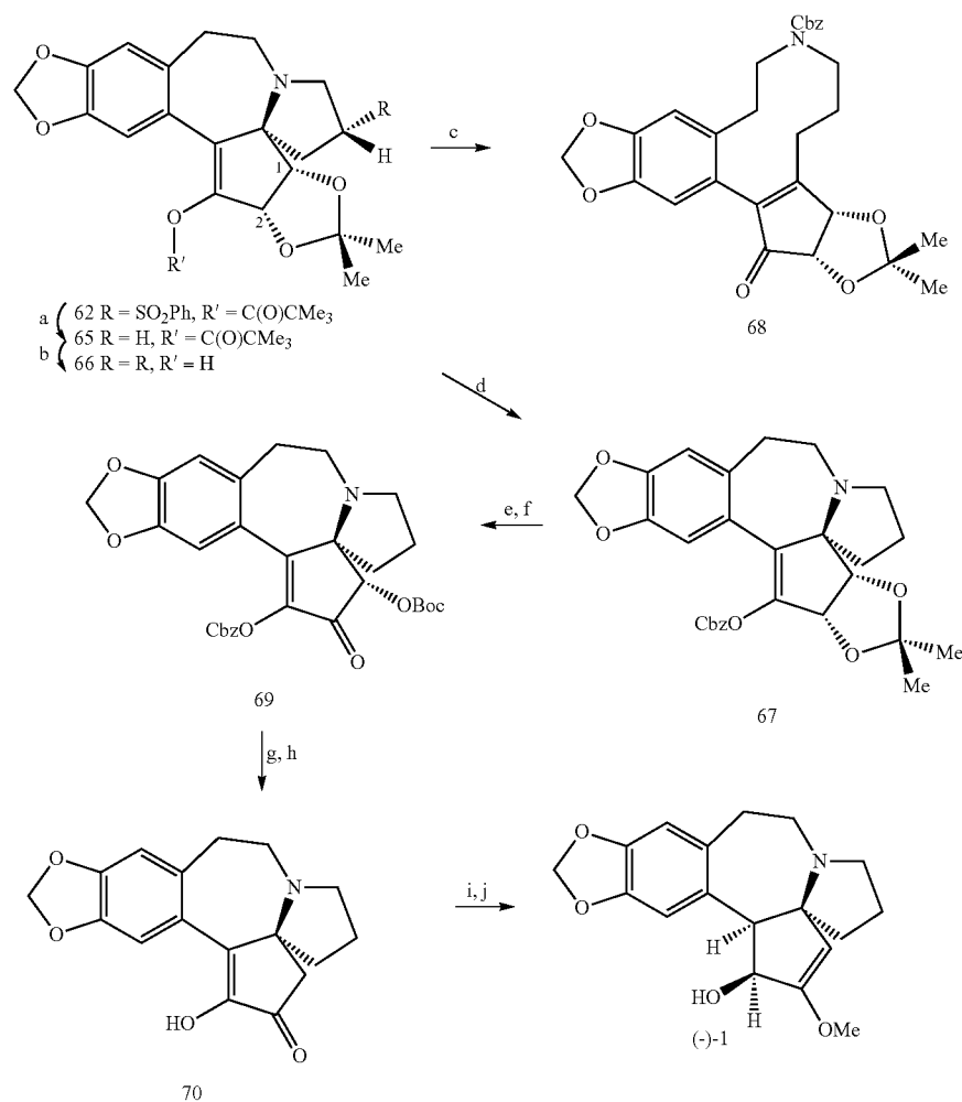
Scheme 12-1.
