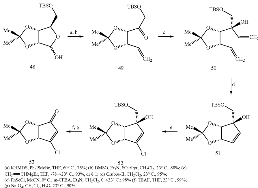
Scheme 8-1.
