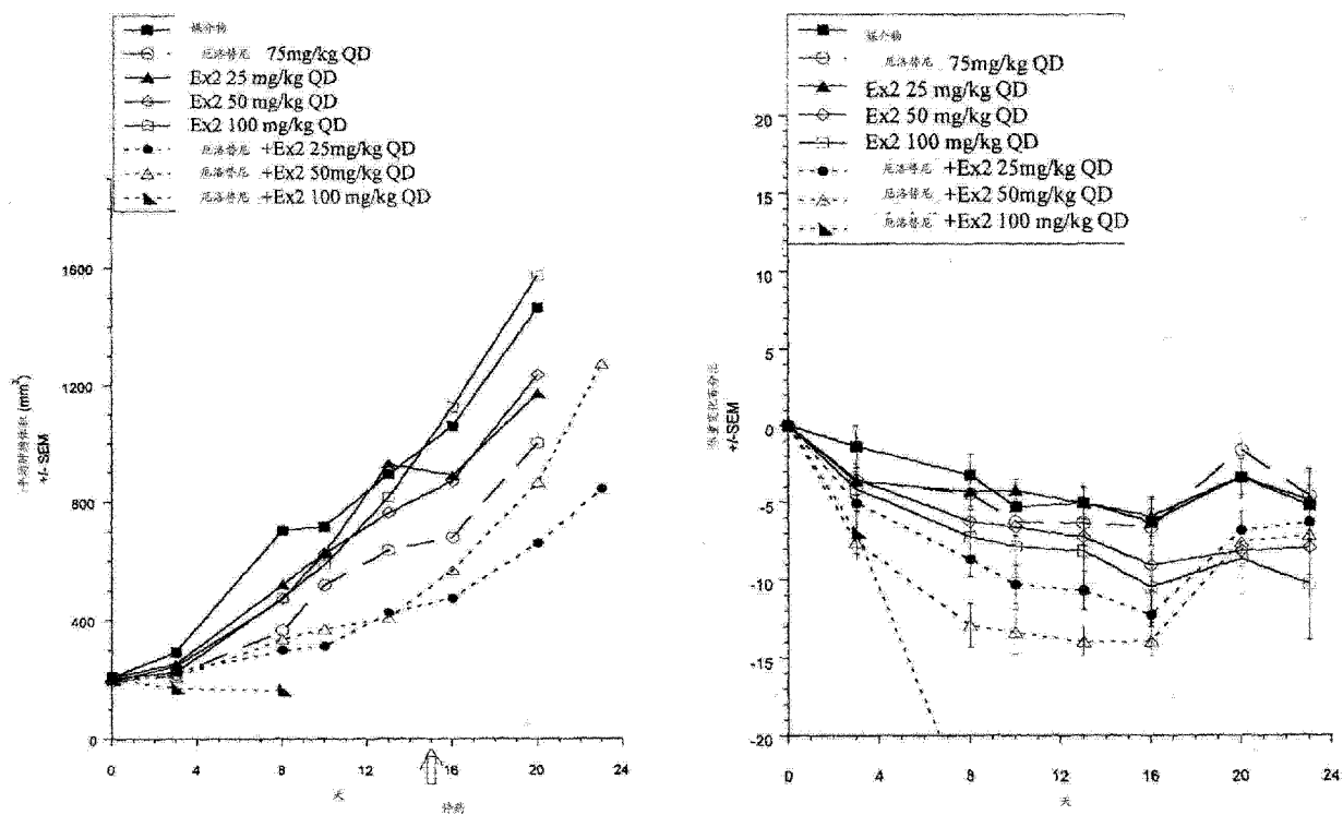
图 1 在 NCI-H2122NSCL 异种移植中的 GDC-0068+ 厄洛替尼
