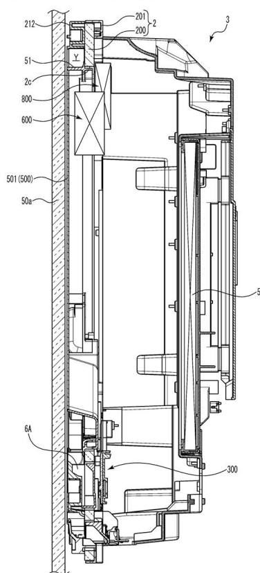
【图 10-4】 A-A 断面图
