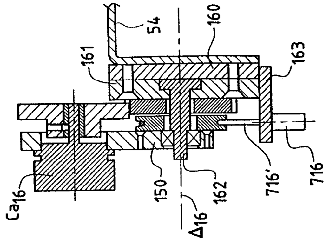
FIG. 3G3 Section U/U
