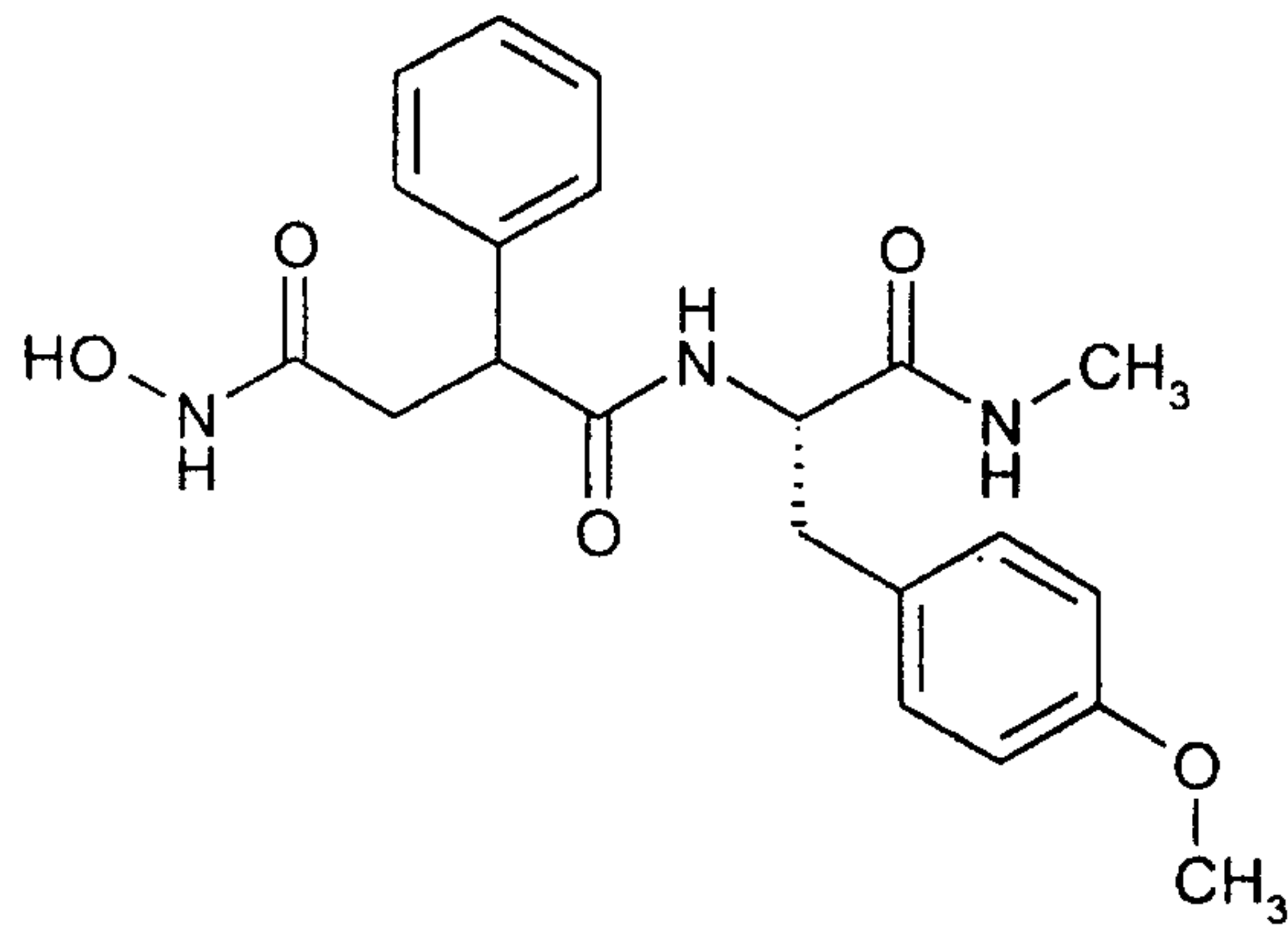
VII IC 50 = 40 nM
