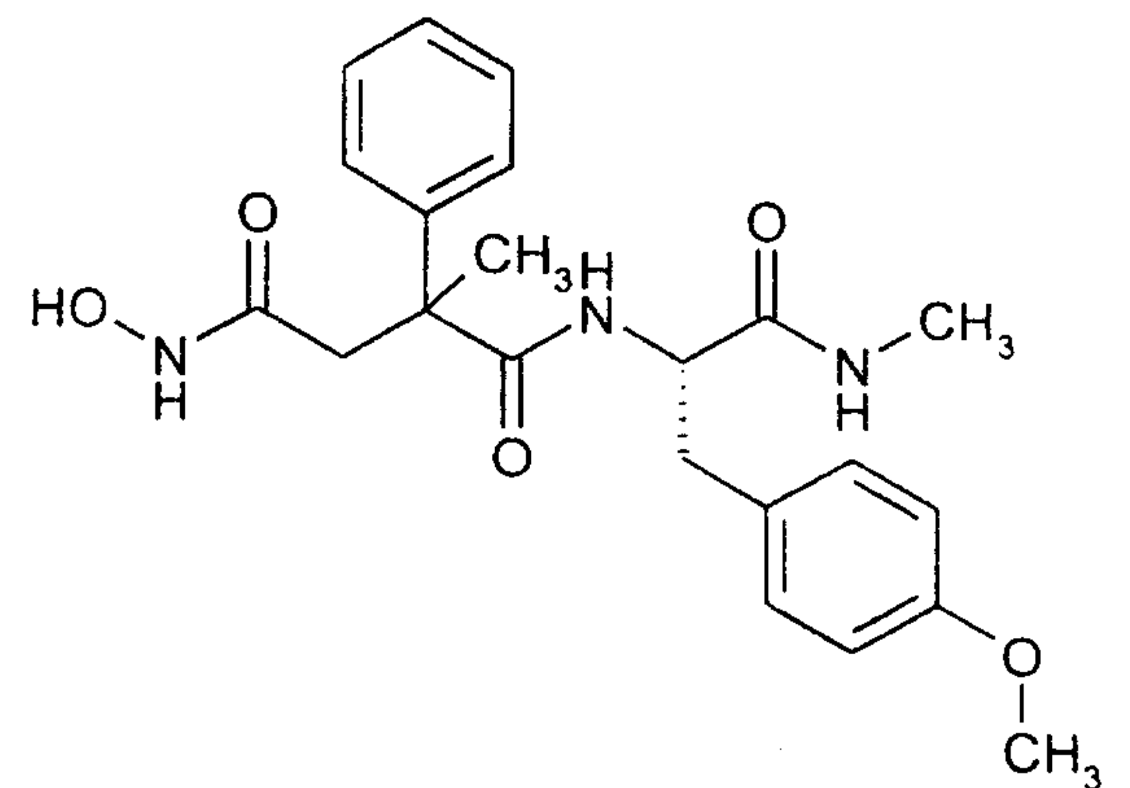
VIII IC 50 = 3800 nM
