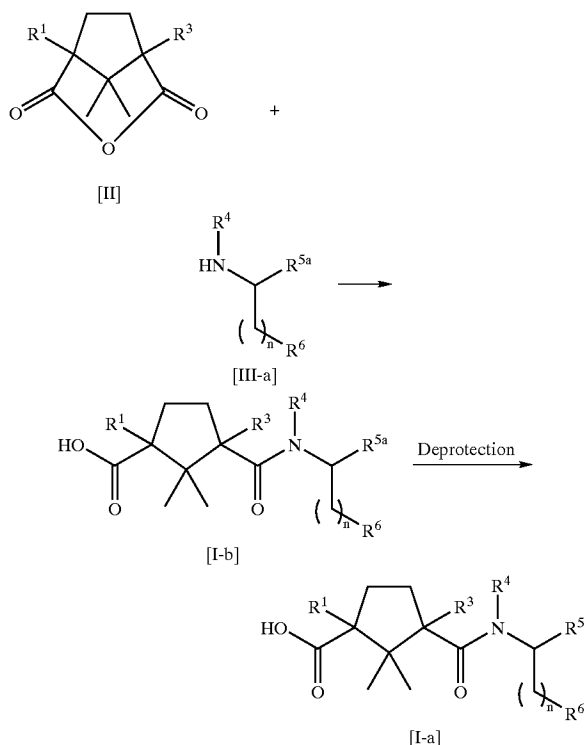
Scheme 1 (Method A):
