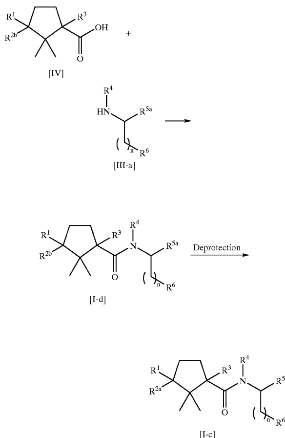
Scheme 2 (Method B):
