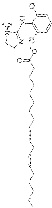
CLX-SX-G77C5-1A, DMSO-16
