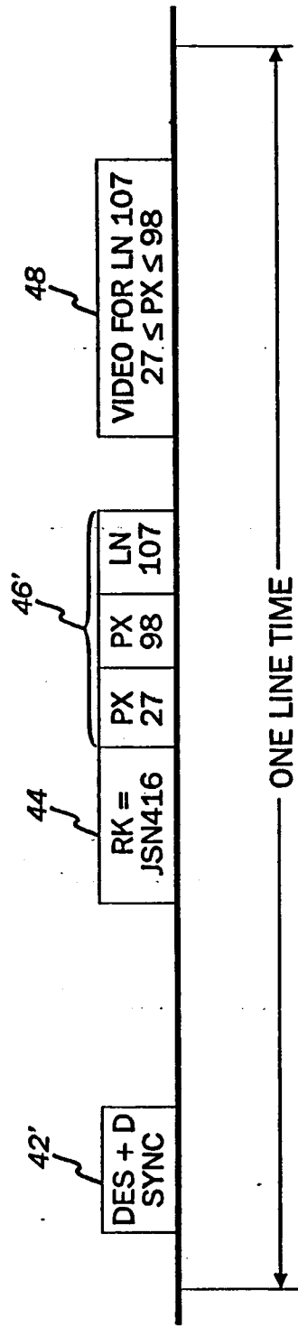
FIG. 3E - DATA ENABLE SEQUENCE PLUS DATA
